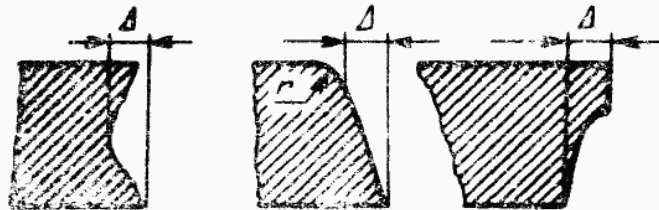
Δ — отклонение поверхности реза от перпендикулярности
